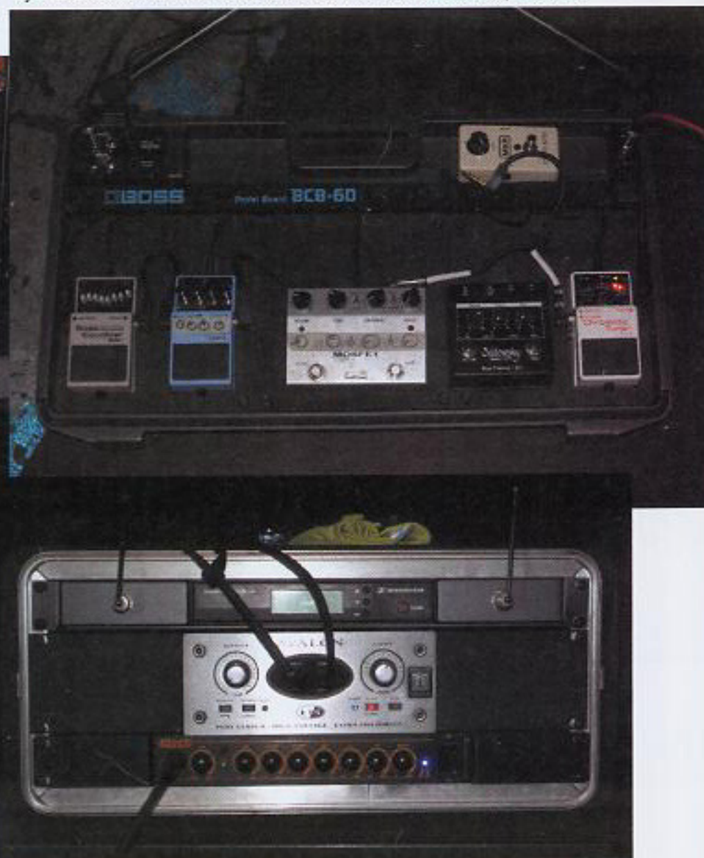
Die Verstärkerabteilung mit Mark Bass F1 und Avalon D.I.
